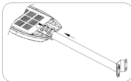
2. 灯臂支架穿到灯体(光伏板面朝上)，螺杆和螺母把青蛙压片和支架固定牢靠。
