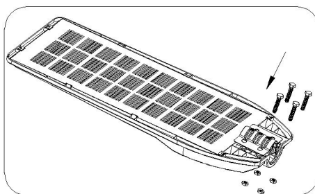
1. 用螺杆和螺母将青蛙压片穿到灯体；
